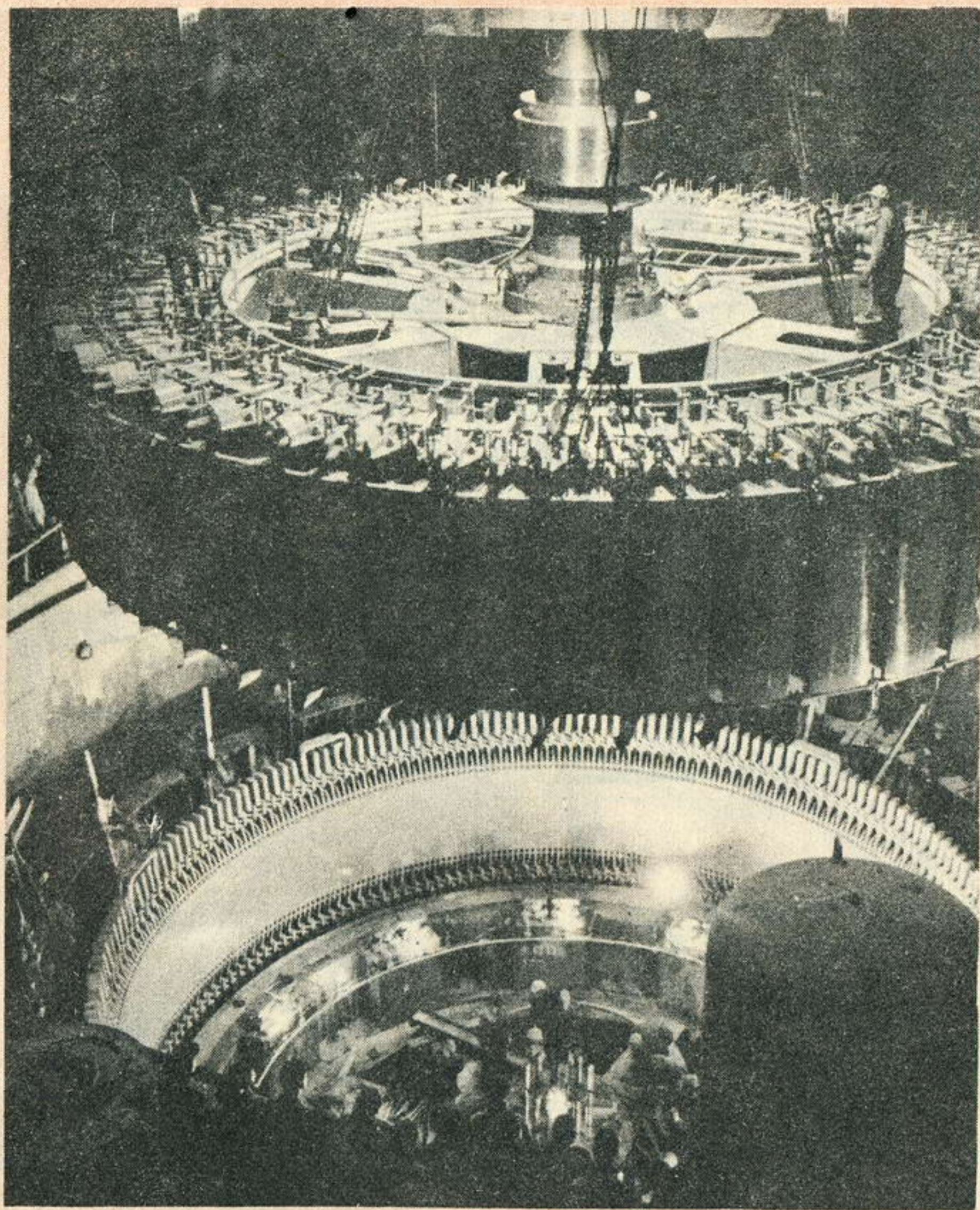
▲哈尔滨电机厂设计制造的三十万瓩水轮发电机组正在新建的大型水电站安装。
